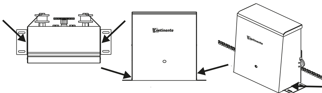
Figura 02: Fixar as bases do Movimentador Deslizante
